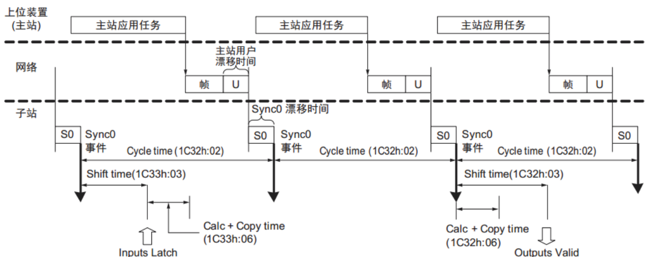
图 7-1 同步时序
