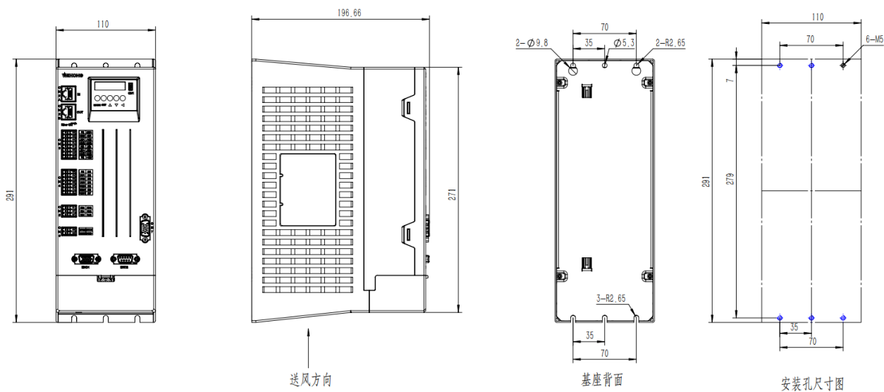
图 2-1 安装尺寸图
