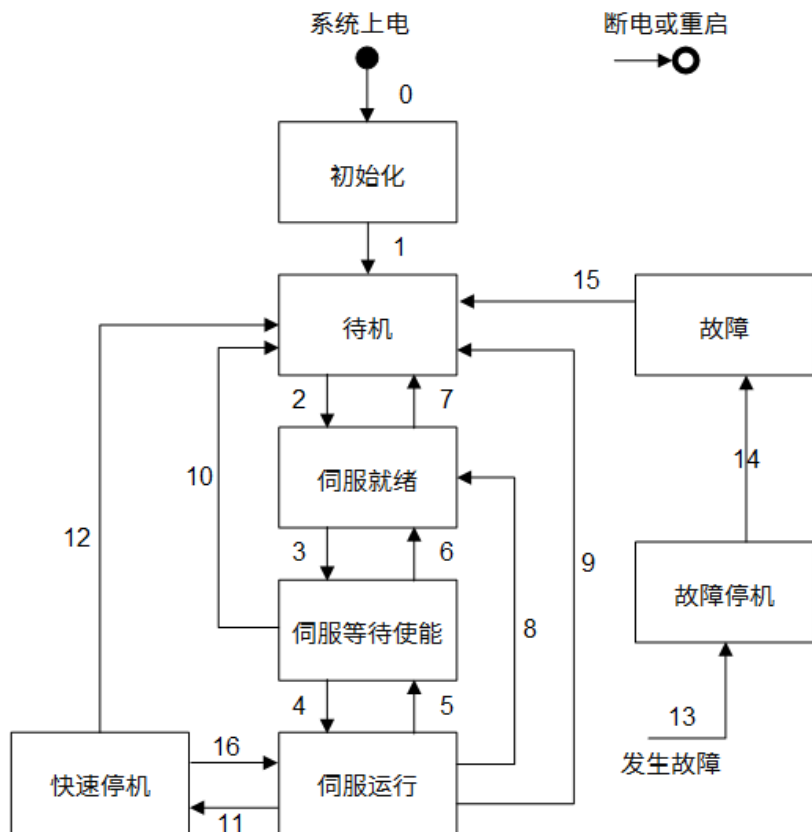
图 8-1 状态迁移图
