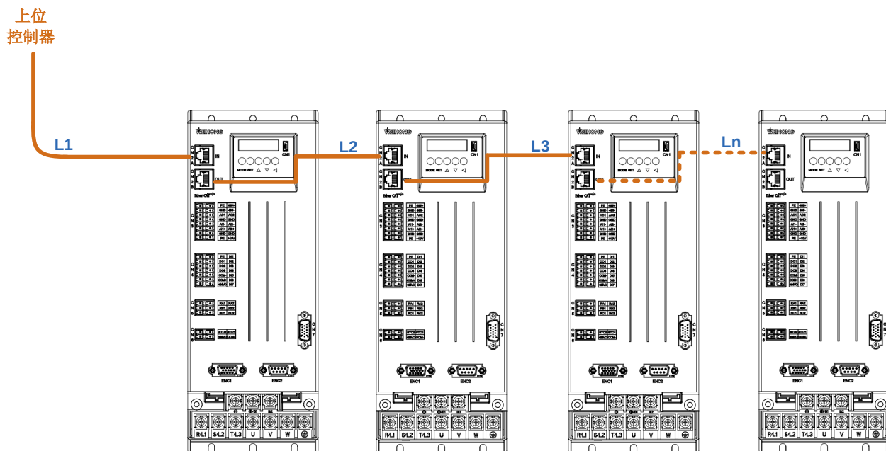
图 3-1 CN2 EtherCAT 通讯接口接线图
