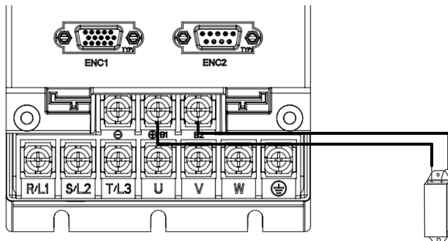
图 3-2 外置再生制动电阻连接示意图
