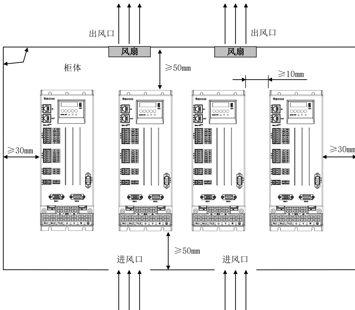
图 2-2 安装空间标准
