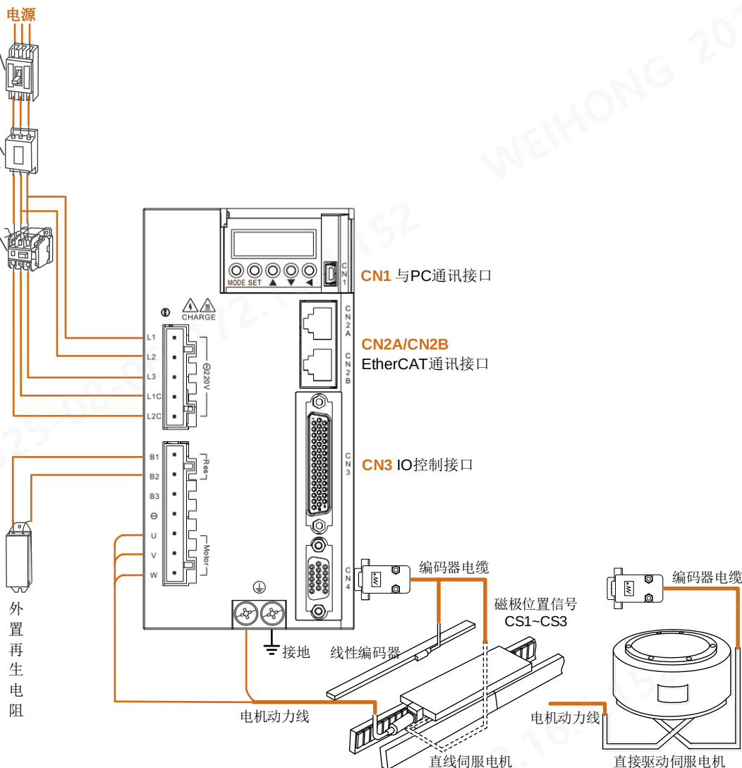
图 1-2 B1L 伺服驱动器与外围设备连接图
