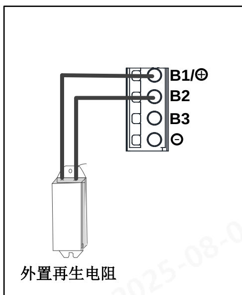
图 3-1 外置再生制动电阻连接图
