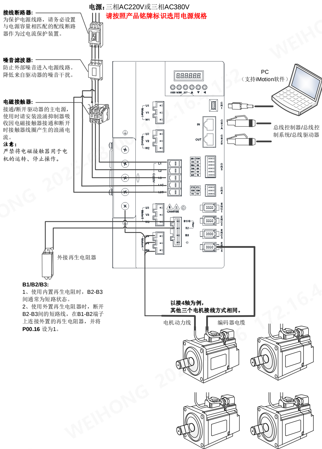
图 1-2 Mini 多轴伺服驱动器与外围设备连接图
