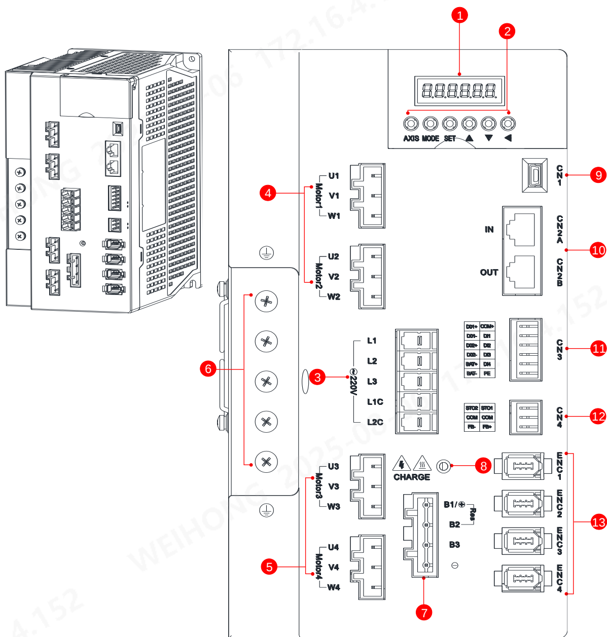
图 1-1 Mini 多轴伺服驱动器组成
