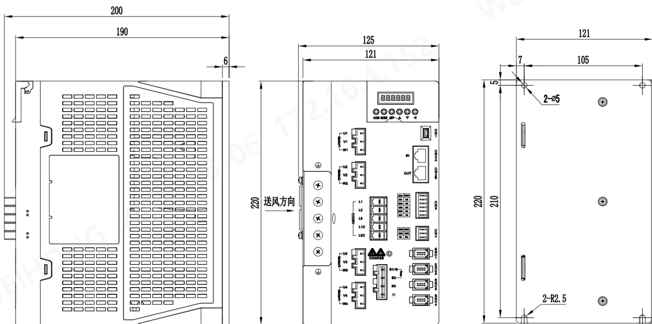
图 2-1 Mini 多轴伺服驱动器安装尺寸图
